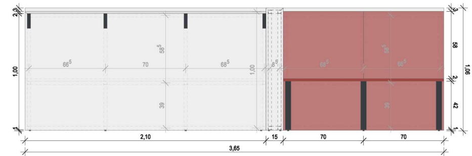
Ansicht Möbel 2er Sitzflächen M 1:20
