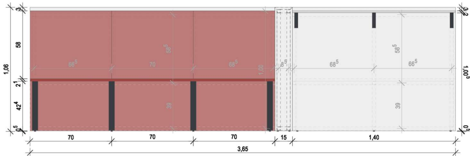
Ansicht Möbel 3er Sitzflächen M 1:20
