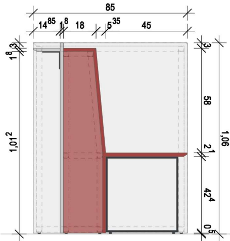
Ansicht Möbel 3er Sitzflächen M 1:20
