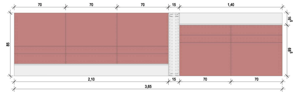
Aufsicht Möbel M 1:20
